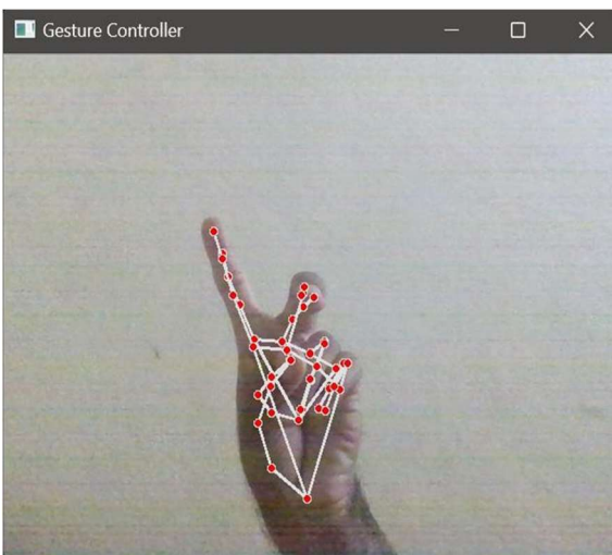
Fig.4. Right Click
