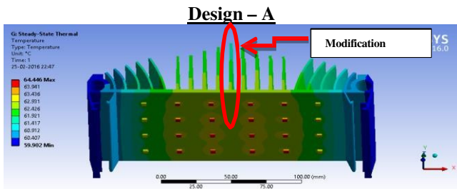
Fig.5 Design-A
